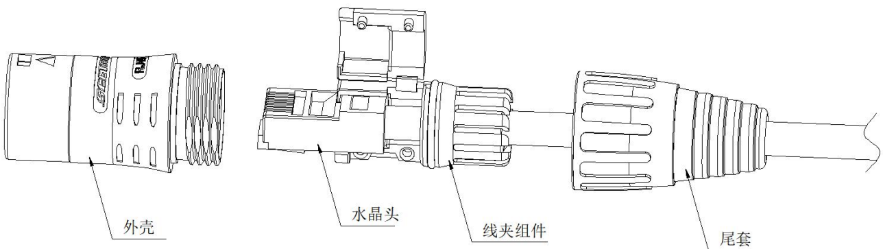
装配示意图
