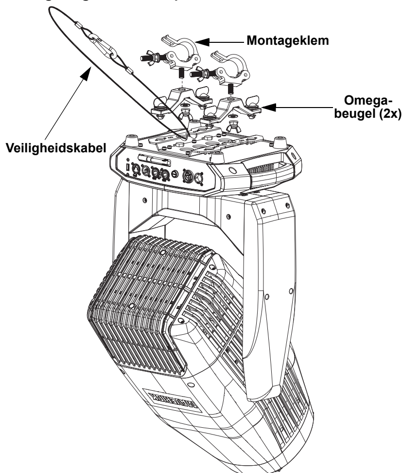
Montage boven het hoofd
